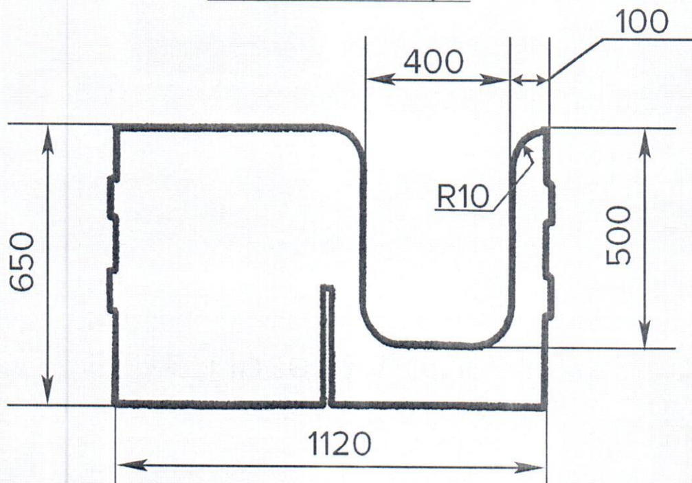
Правый борт
